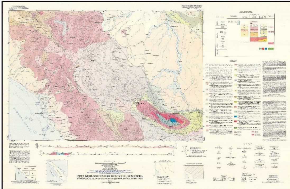
Gambar 2. Peta Geologi
