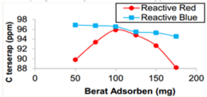
Gambar 3. Kurva Hubungan Antara Berat Adsorben Dengan Konsentrasi Terserap Larutan Zat Warna Reactive Red Dan Reactive Blue Menggunakan AACB
