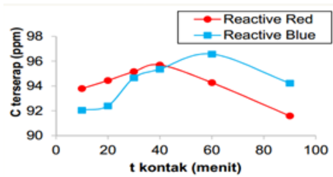
Gambar 2. Kurva Hubungan Antara Waktu Kontak Dengan Konsentrasi Terserap Larutan Zat Warna Reactive Red Dan Reactive Blue Menggunakan AACB
