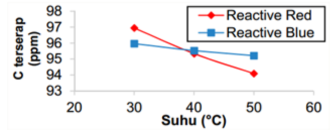
Gambar 4. Kurva Hubungan Antara Suhu Dengan Konsentrasi Terserap Larutan Zat Warna Reactive Red Dan Reactive Blue Menggunakan AACB
