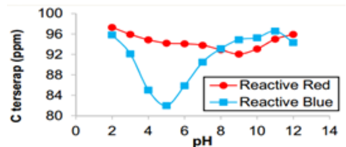
Gambar 1. Kurva Hubungan Antara pH Dengan Konsentrasi Terserap Larutan Zat Warna Reactive Red Dan Reactive Blue Menggunakan AACB
