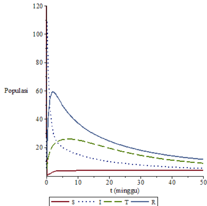
Gambar 3. Solusi Sistem (1) saat \mathcal{R}_0 > 1
