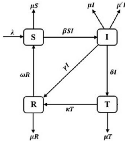
Gambar 1. Diagram transfer model SITRS pada penyebaran diare
