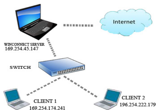
Gambar 1. Topologi Jaringan
