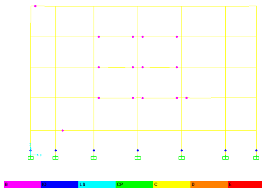
Gambar 9. 2D Sendei Plastis Push Y Step 8 (Data Pribadi Hasil Analisis SAP 2000, 2020)
