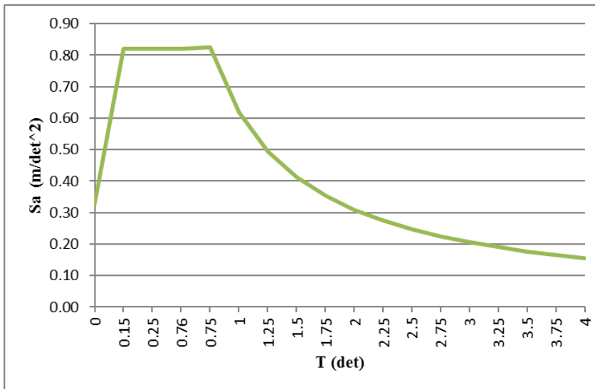
Gambar 4. Grafik Respon Spktrum (Data Pribadi Hasil Analisis, 2020)
