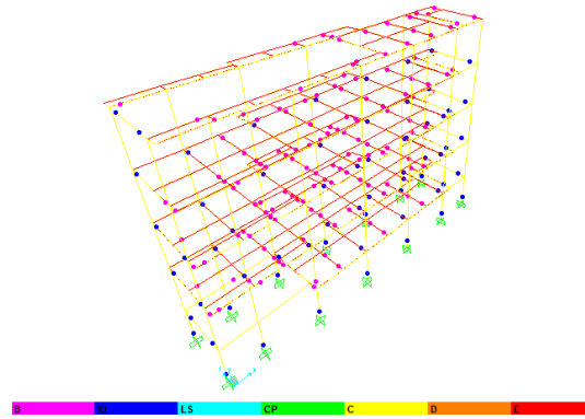
Gambar 10. 3D Sendei Plastis Push Y Step 8 (Data Pribadi Hasil Analisis SAP 2000, 2020)
