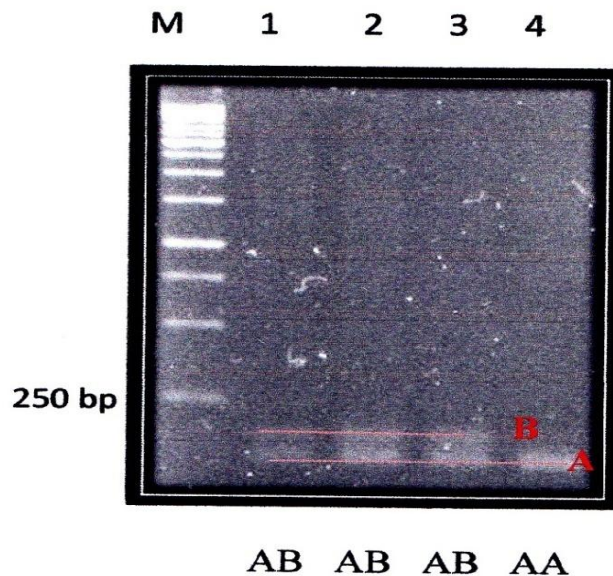
Gambar 2. Pola pita lokus CMO211
