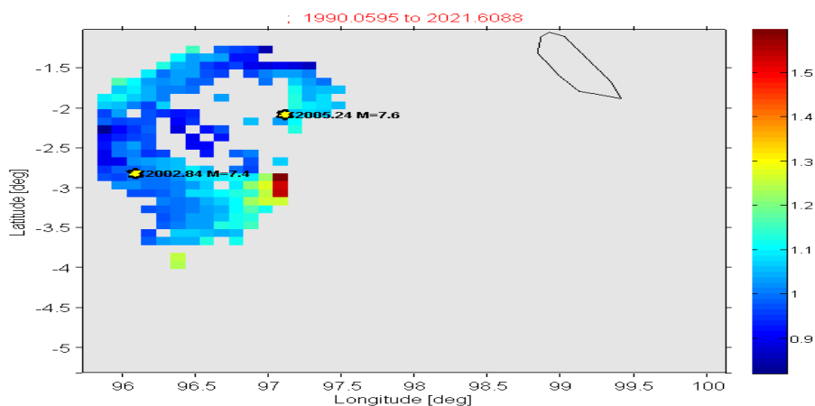
Gambar 6. Sebaran b-value Wilayah Sumatera Utara
