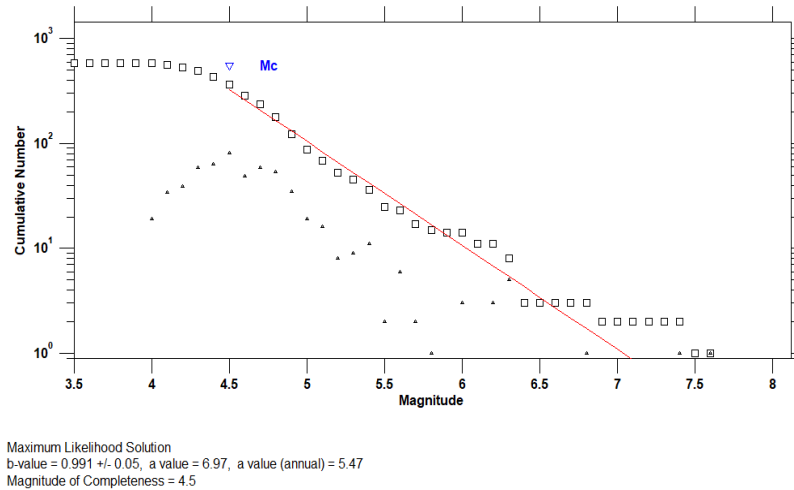
Gambar 4. Distribusi frekuensi - magnitudo wilayah Sumatera Utara (1990-2021).
