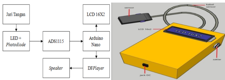
Gambar 3. Blok Diagram Alir Penelitian dan Rangkaian Alat Ukur Kadar Gula Darah
