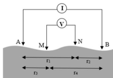
Gambar 3. Susunan elektroda metode geolistrik resistivitas
