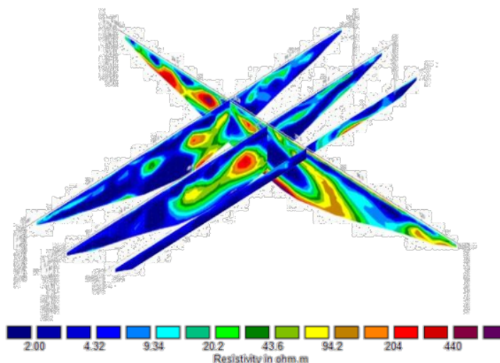
Gambar 9. Hasil korelasi penampang litologi bawah permukaan pada lintasan 1–4
