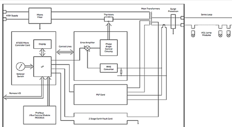
Gambar 1. Blok Diagram CCR ke Instalasi PAPI
