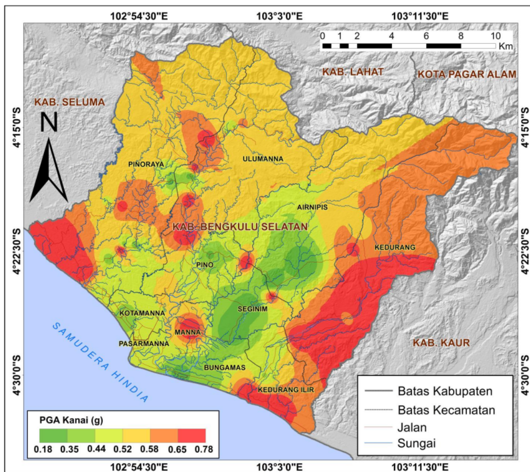
Gambar 4. Peta nilai PGA berdasarkan sumber gempa 100 tahun.
