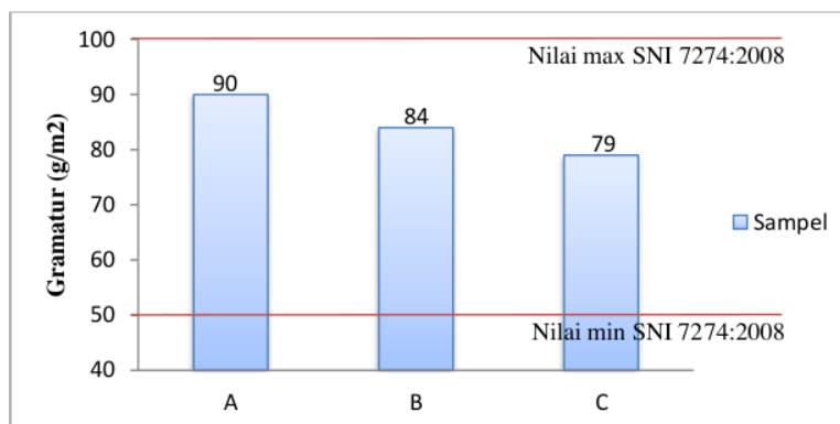
Gambar 4. Grafik Hasil Uji Gramatur Kertas
