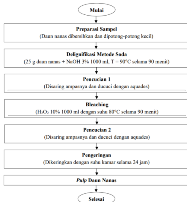
Gambar 1. Diagram Alir Tahap Pembuatan Pulp Daun Nanas
