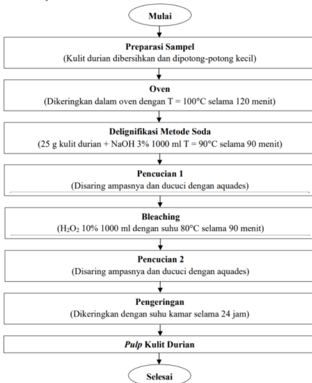
Gambar 2. Diagram Alir Tahap Pembuatan Pulp Kulit Durian
