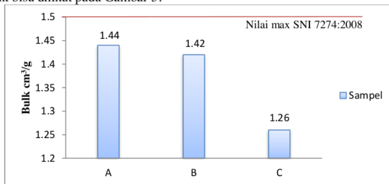
Gambar 5. Hasil Uji Bulk Kertas
