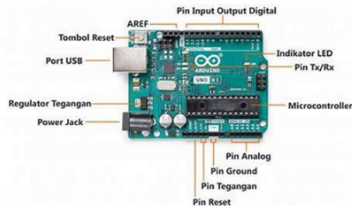
Figure 1. Arduino uno
