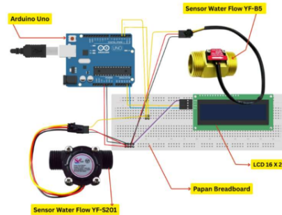
Gambar 5. Perancangan Perangkat Keras (Hardware)
