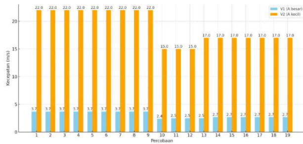
Gambar 8. Diagram Perbandingan Nilai Kecepatan Antar Penampang
