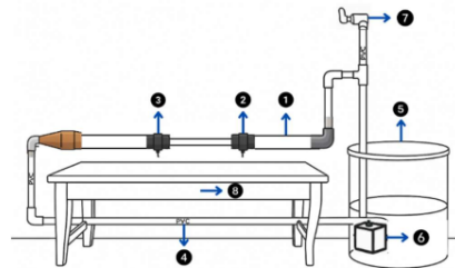
Gambar 6. Desain Prototipe Alat Peraga
