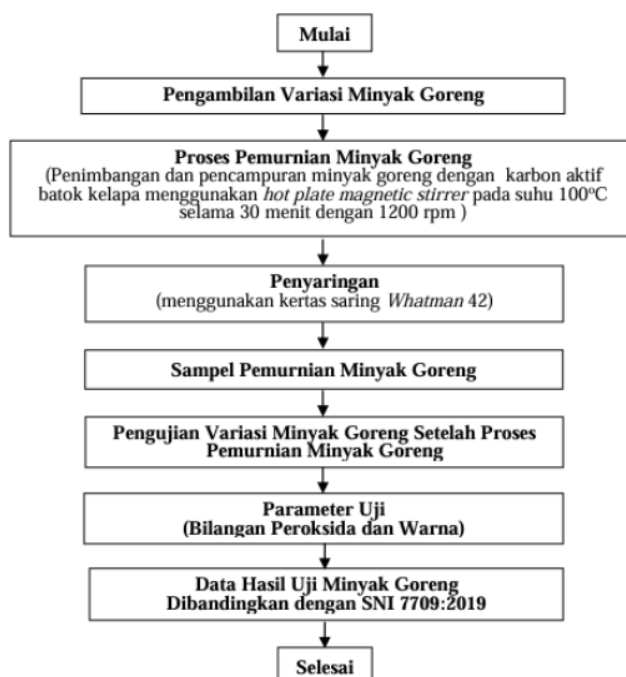
Gambar 3. Diagram Alir Tahap Pengujian Minyak Goreng Bekas Setelah Pemurnian Minyak Goreng
