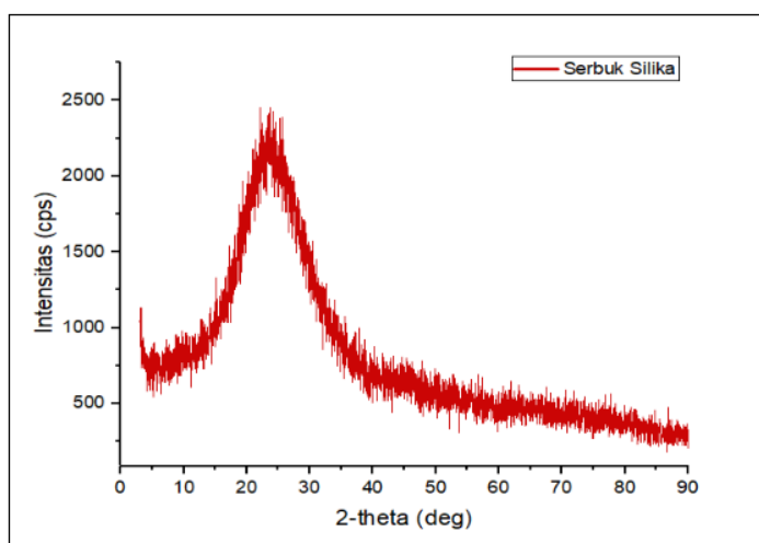
Gambar 2. Difraktogram serbuk silika ( \text{SiO}_2 ) hasil ekstraksi.
