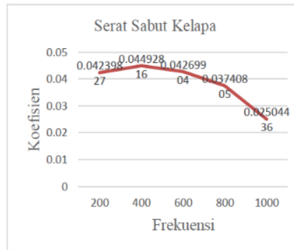
Gambar 4. Grafik Serat Sabut Kelapa
