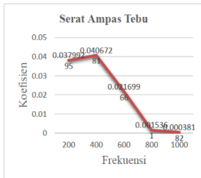
Gambar 3. Grafik Serat Ampas Tebu
