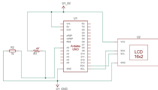
Gambar 1. Skematik rangkaian luxmeter dengan sensor LDR
