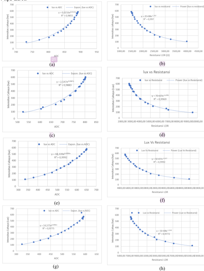
Gambar 1 Sebaran data ADC dan Resistensi terhadap lux serta model regresi eksponensial (a) GL5506, (c) GL5528, (e) GL5537, (g) GL5539 dan regresi power (b) GL5506, (d) GL5528, (f) GL5537, (h) GL5539 Berdasarkan grafik sebaran data ADC terhadap nilai lux {gambar 1(a); 1(c); 1(e) dan 1(g)} yang ditunjukkan pada model regresi eksponensial, nilai R^2 atau koefisien determinasi keempat tipe LDR
