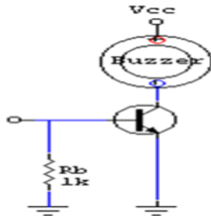
Gambar 4. Rangkaian Penguat Alarm
